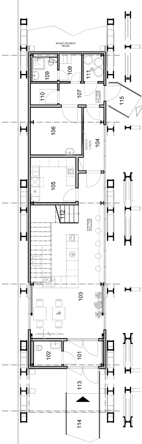
PÔDORYS 1. NP 9 MIEST NA SEDENIE
