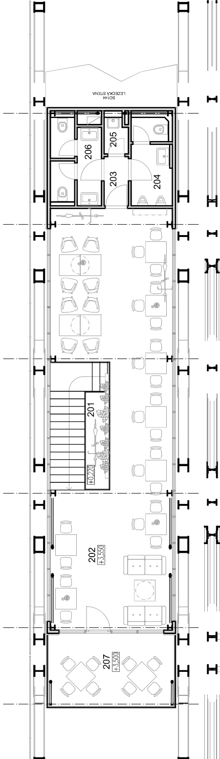
PÔDORYS 2. NP 42 MIEST NA SEDENIE
