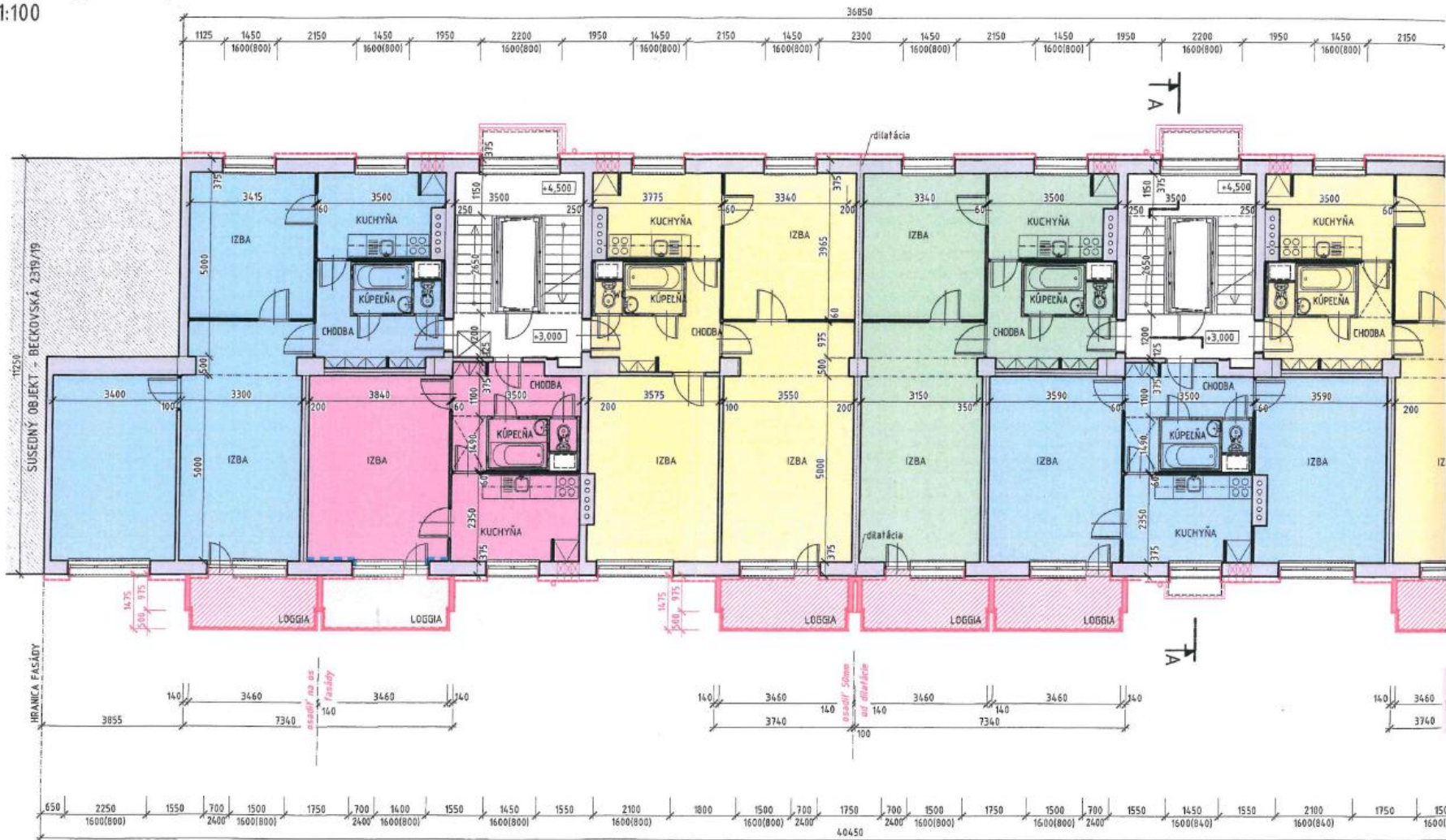
Pôdorys typického podlažia
