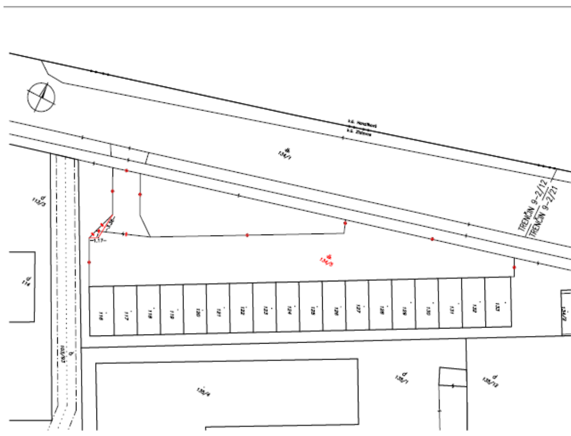
Geometrický plán č. 48035637-097-23 na oddelenie pozemku C KN p.č. 134/5 o výmere 335 m 2 .
