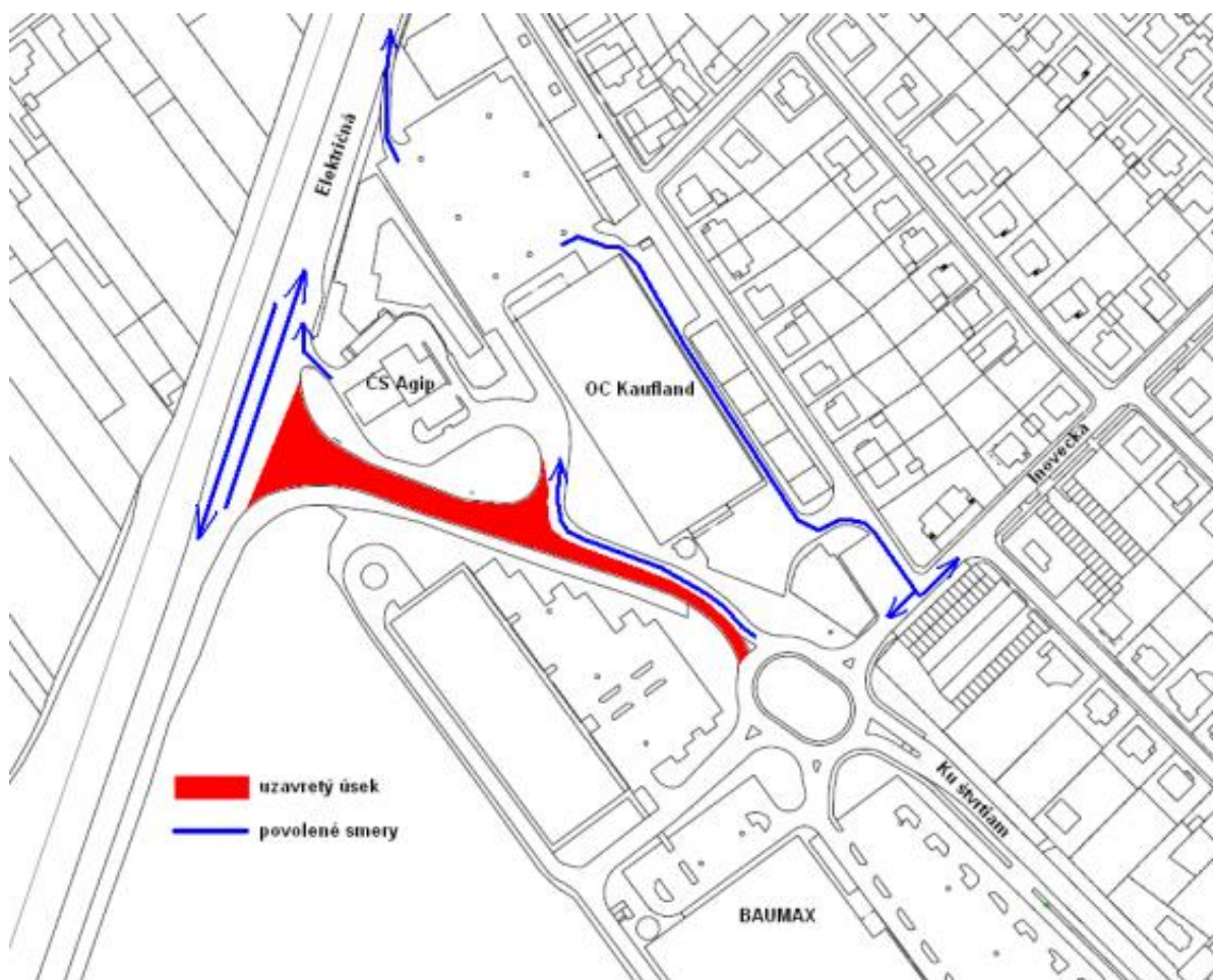
organizácia dopravy počas výstavby kruhového objazdu pri Agipe
